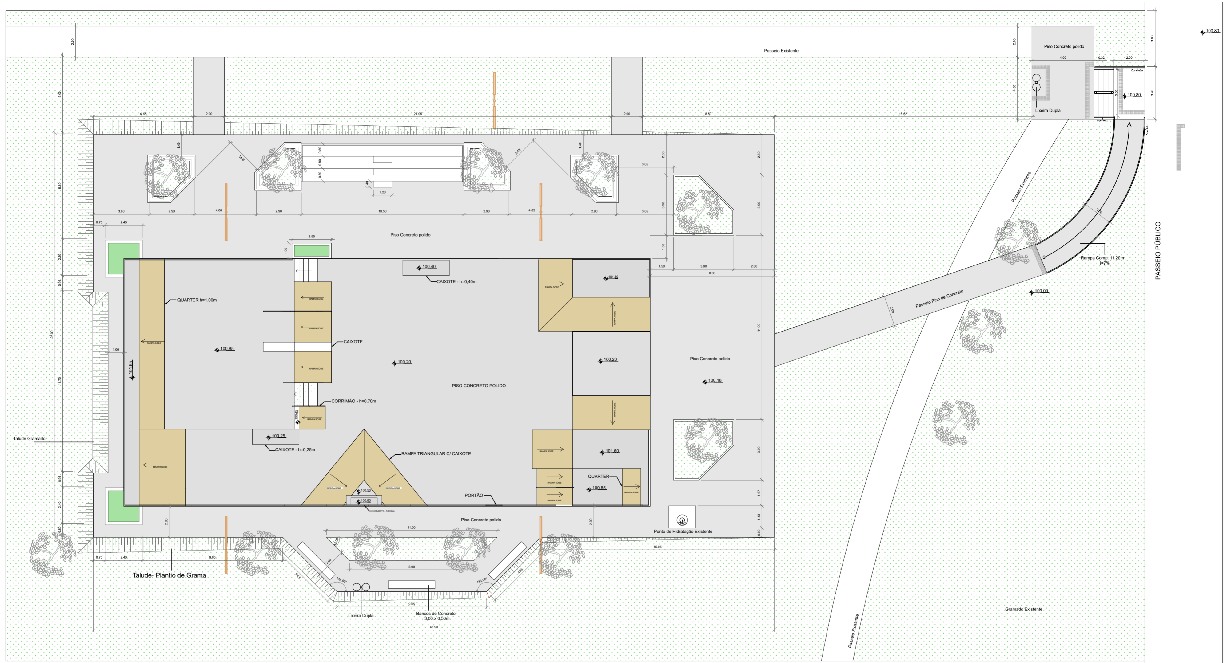
IMPLANTAÇÃO Esc.: 1/150
